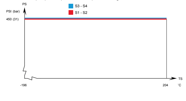
DOC30 – Graphique de pression/température agrément UL
